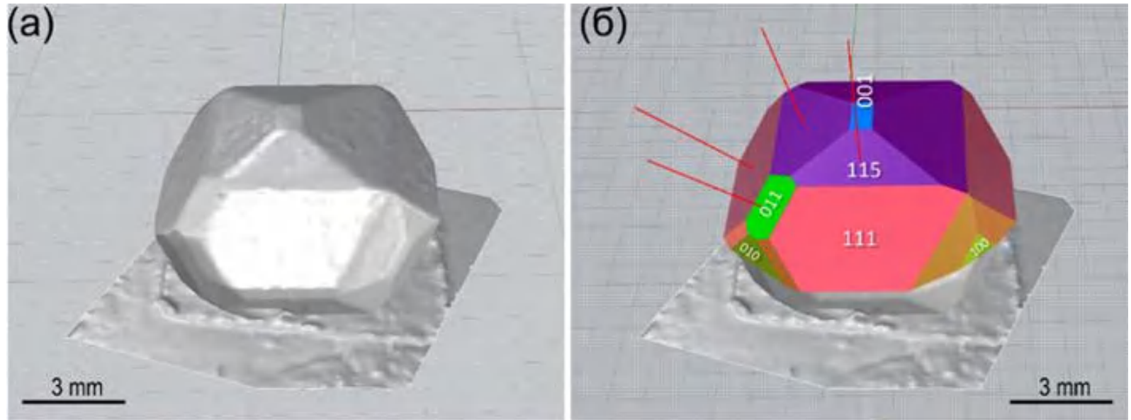
Реконструкція секторів росту: (а) – 3D скан кристалу (хмара точок), (б) – векторизована модель граней та відповідні нормалі.
